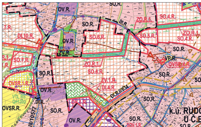
Výřez koordinačního výkresu územního plánu z roku 2008, plynovody jsou zakresleny zelenou barvou jako stav, vč. bezpečnostního pásma
